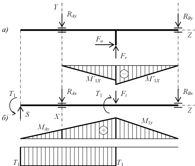
Рисунок 5 — Схема нагружения вала редуктора: а — в вертикальной плоскости; б — в горизонтальной плоскости
