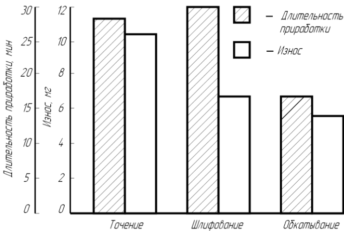
Рисунок 25 — Зависимость длительности обработки и износа от вида обработки
